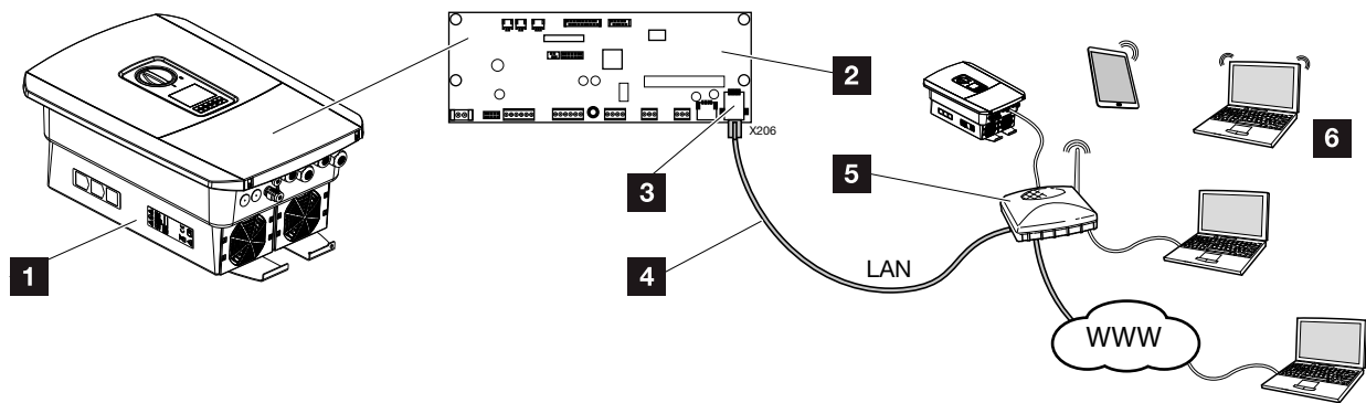
Abb. 27: Anschluss Kommunikation
